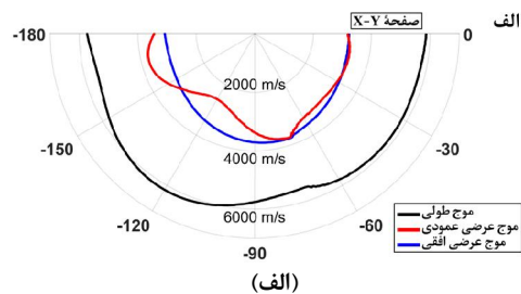
شکل ۷- منحنی گندی ماتریس سختی حاکم بر جوش فریتی-آستنیتی
