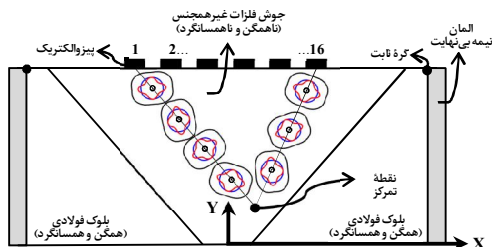
شکل ۶- تقسیم بندی فاصله بین پیزوالکتریک‌ها تا نقطه تمرکز
