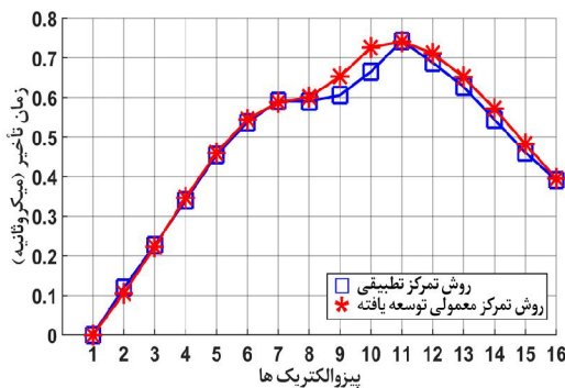
شکل ۱۴- زمان تأخیر محاسبه شده به روش تمرکز تطبیقی و روش تمرکز معمولی توسعه یافته (جوش فریتی-آستنیتی)
