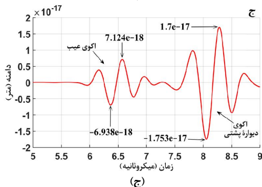
شکل ۱۸- سیگنال دریافتی از جوش فریتی-آستنیتی؛
